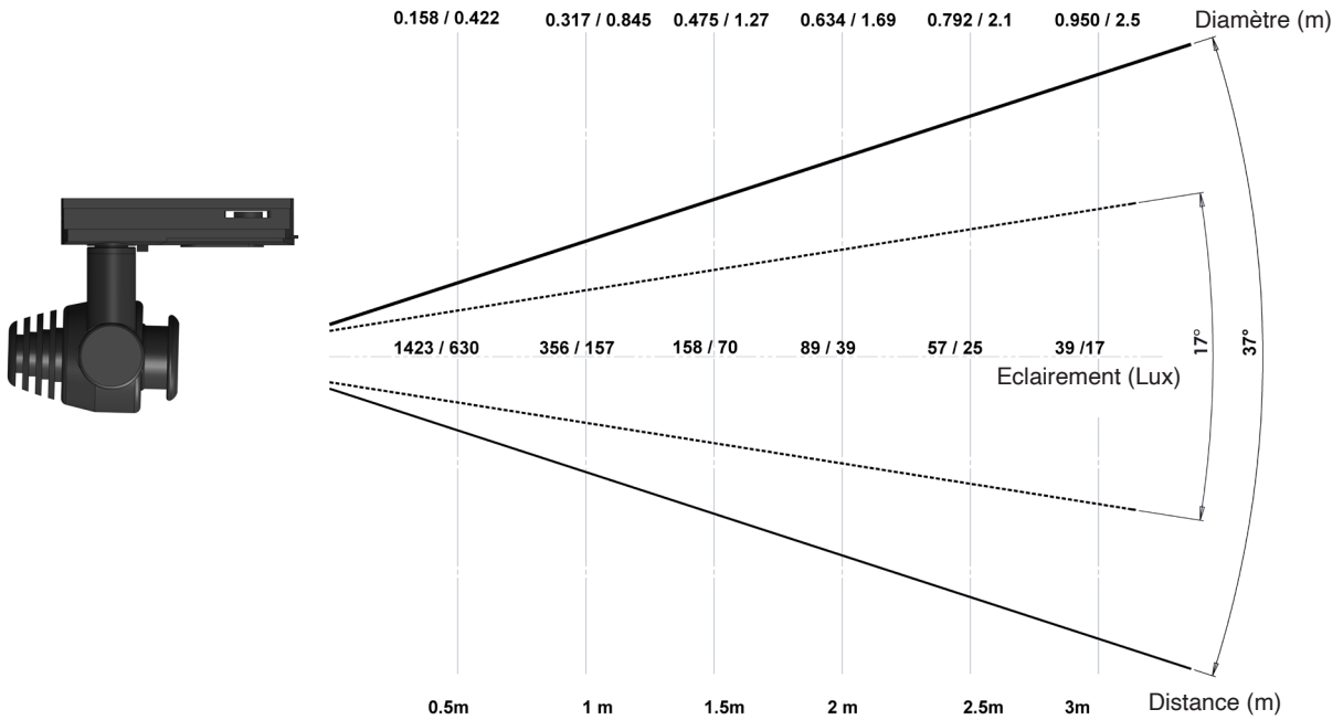
MOOVEO HR 3000K 17° à 37°
